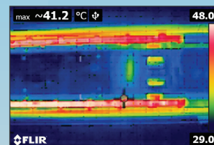
Termografski prikaz svetila v uporabi.
